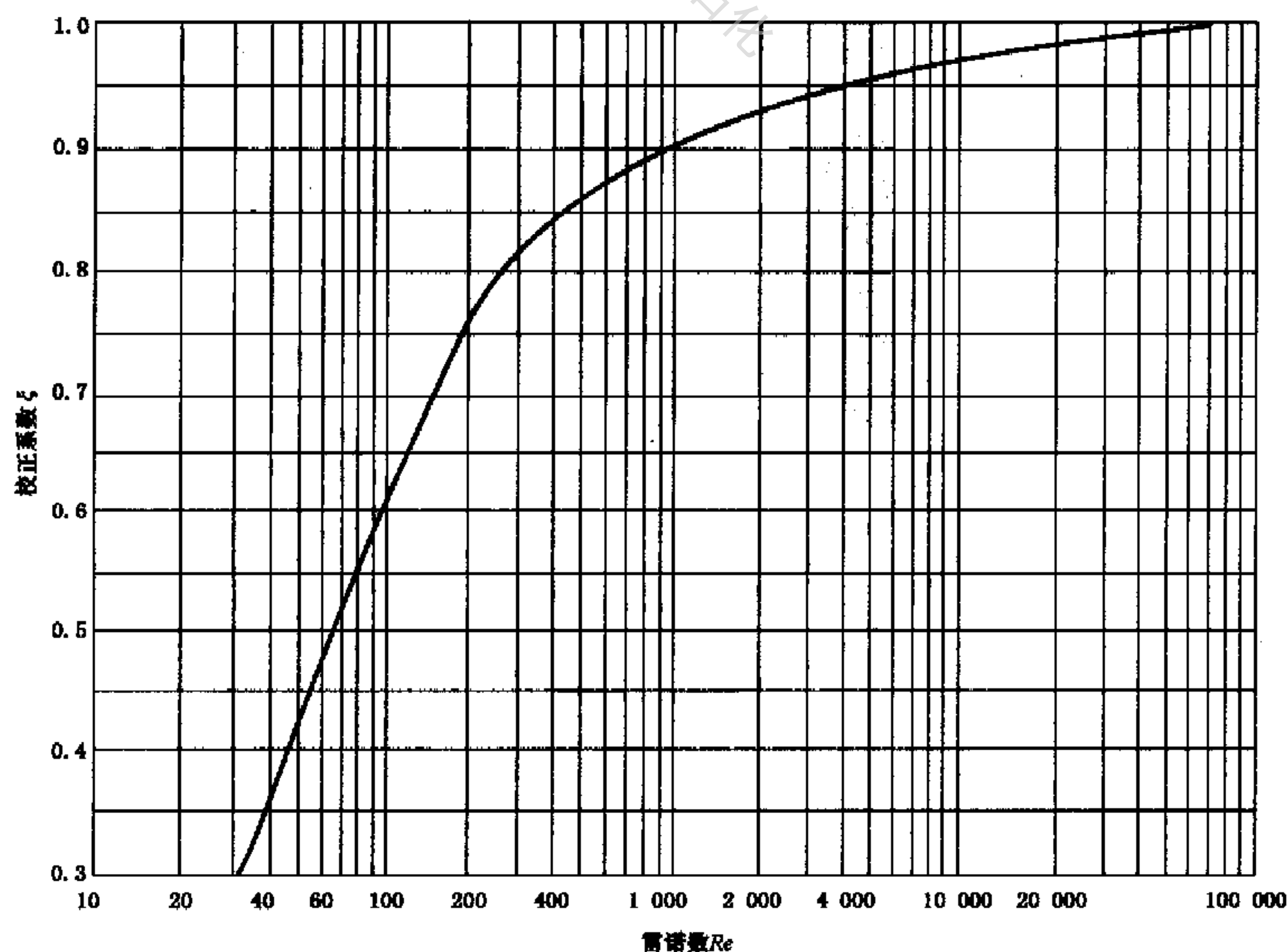
图 A.2 液体动力黏度校正系数 \xi
